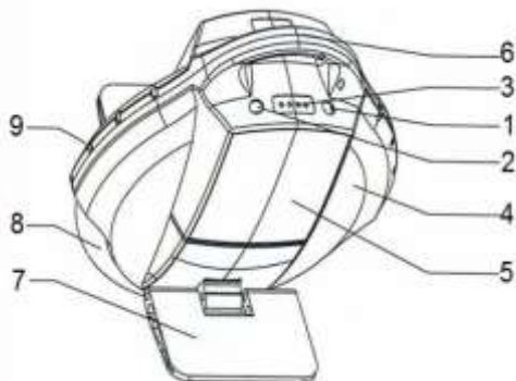
Рисунок 1. Основные элементы моноколеса Sunwheel
